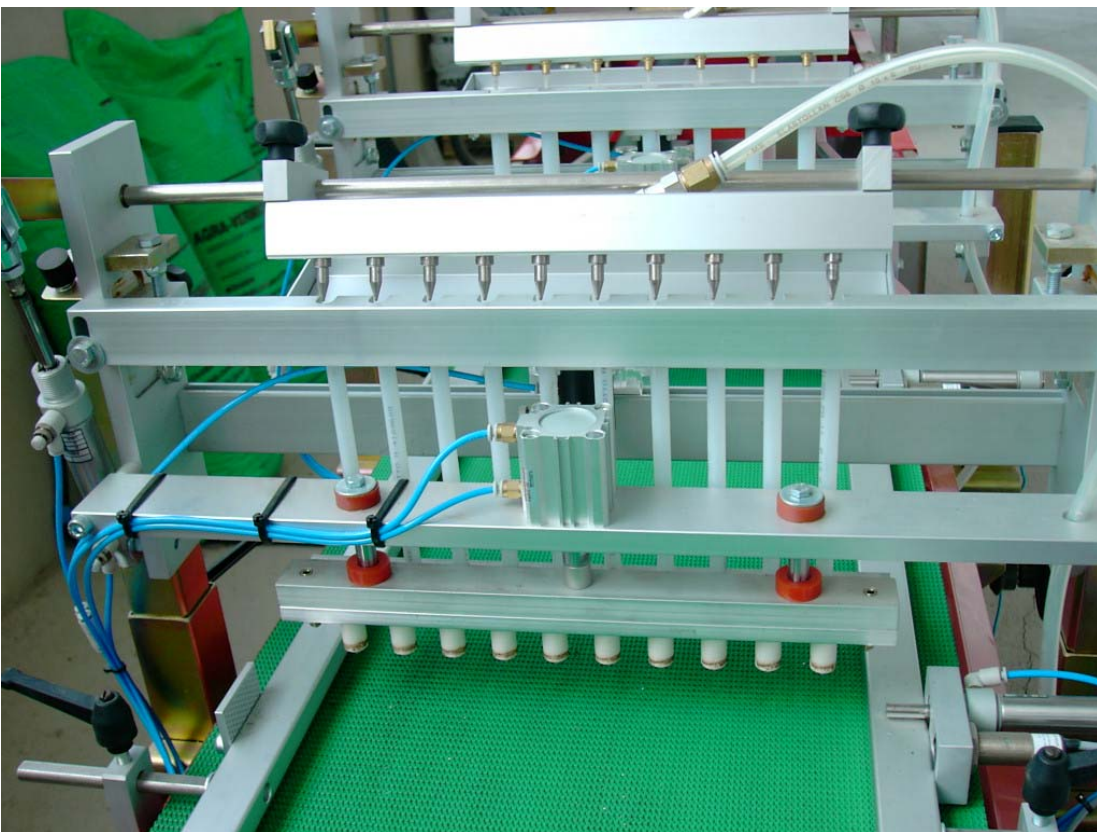
Sowing head
